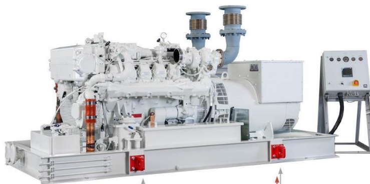
Sicherheitssystem mit Notstopp-Funktion für Diesel Motoren AHD 514 S
